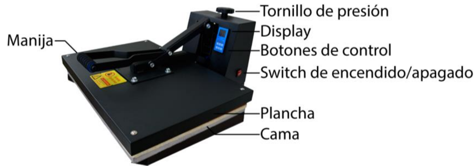
Figura 1. Equipos STM-46S
